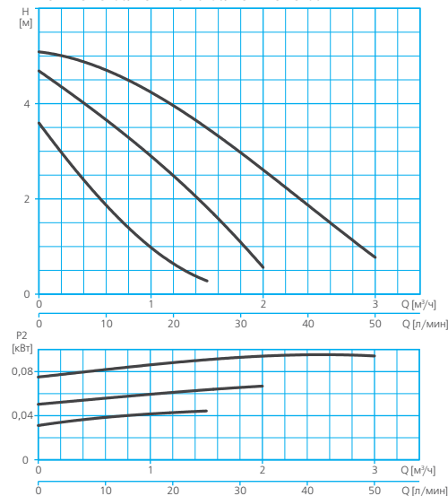
RSAN-S 15-60/ RSAN-S 20-60/ RSAN-S 25-60
