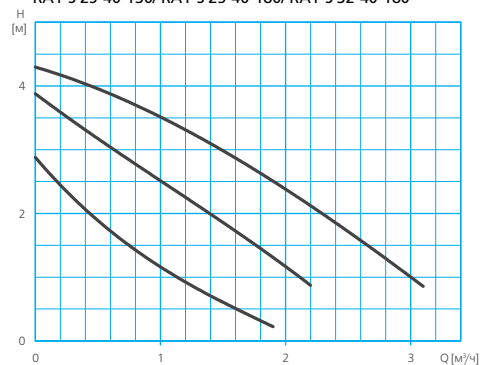
RA1-S 15-40-130/ RA1-S 20-40-130/ RA1-S 20-40-180/ RA1-S 25-40-130/ RA1-S 25-40-180/ RA1-S 32-40-180
