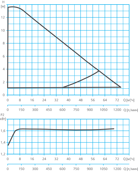
NMT F 80 / NMT F 100
